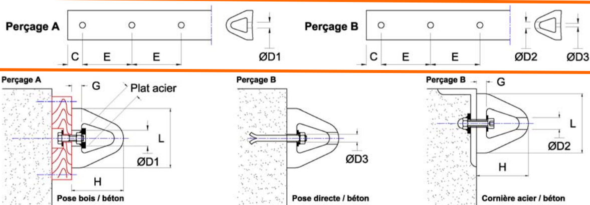
Les schémas de montage ci-dessus ne sont que des exemples, chaque application particulière pouvant donner lieu à une adaptation propre de l'ensemble à protéger
